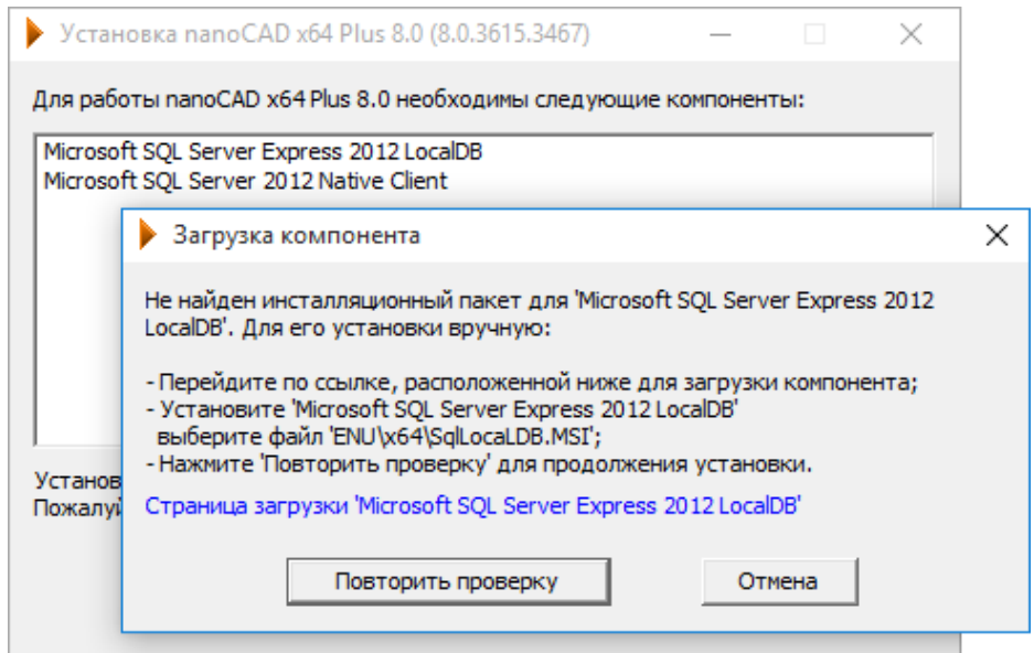
Загрузка компонента
